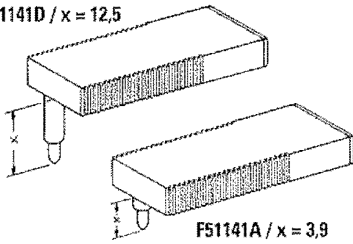
F51141D / x = 12,5
